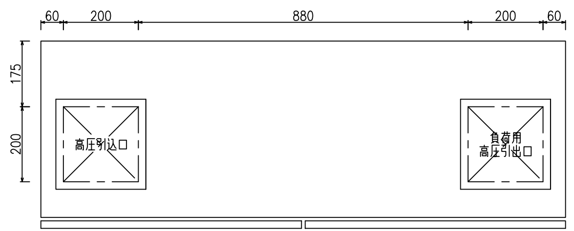
A-A'断面図
