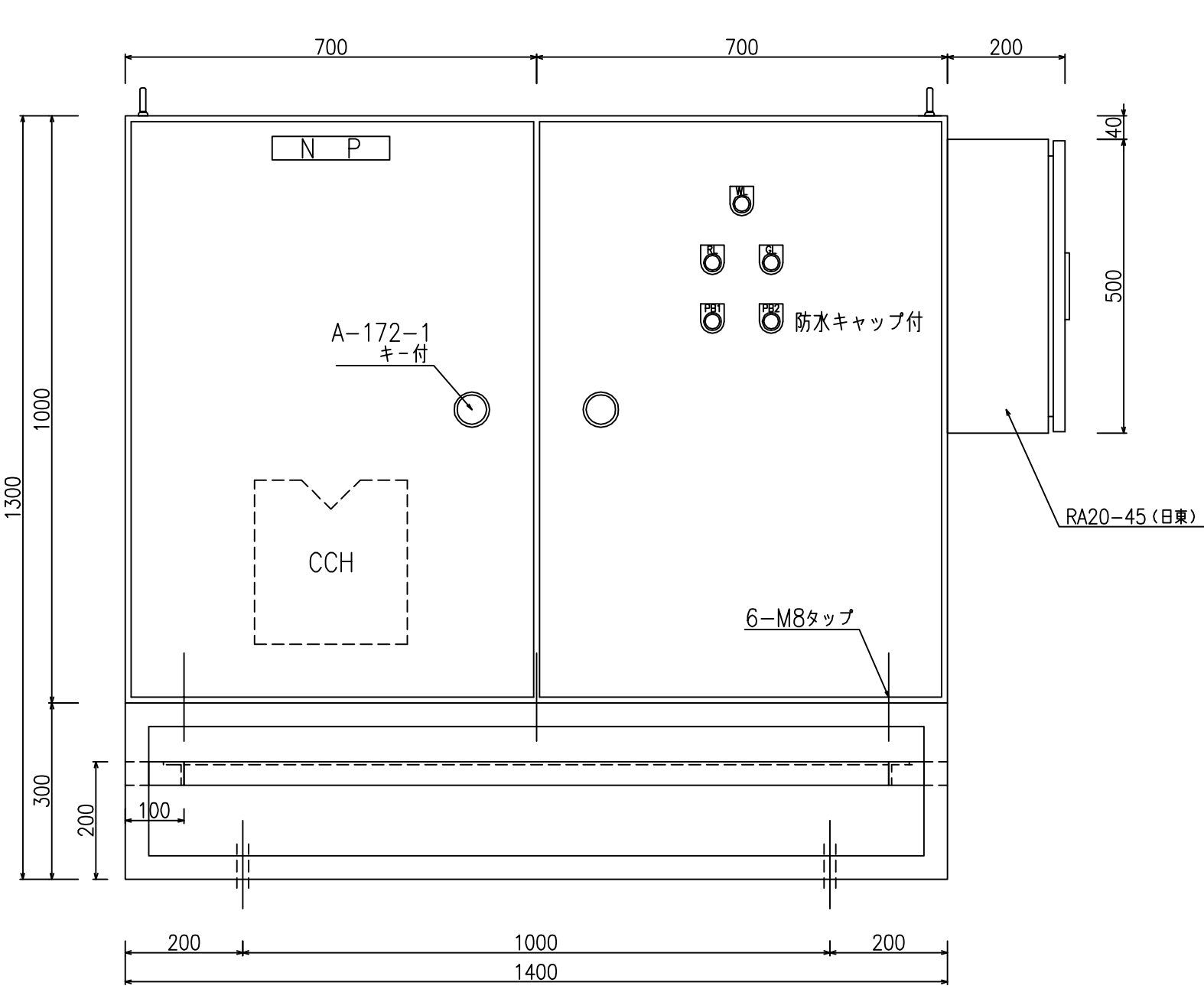
正面図
