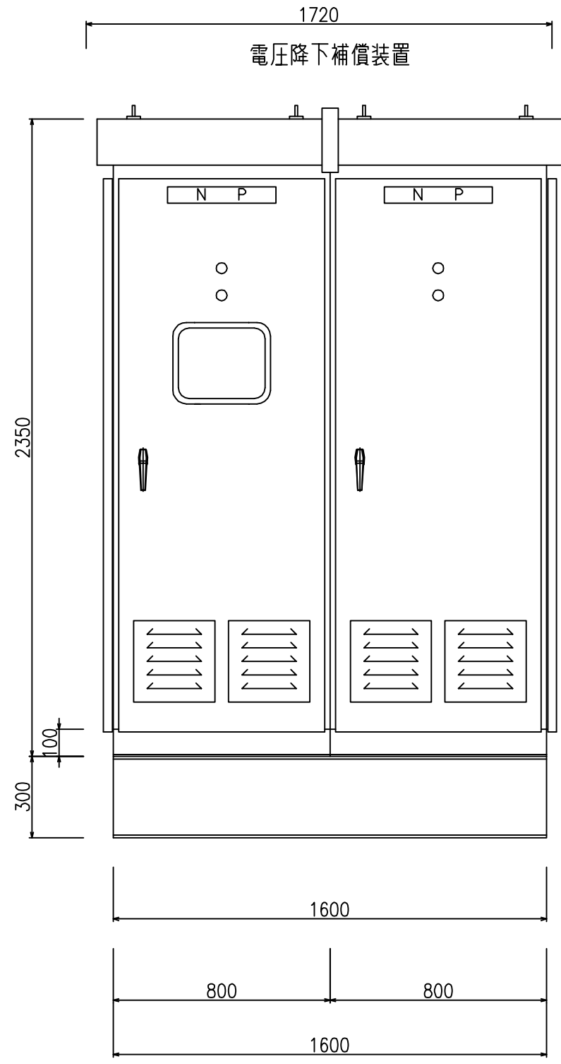
正面図
