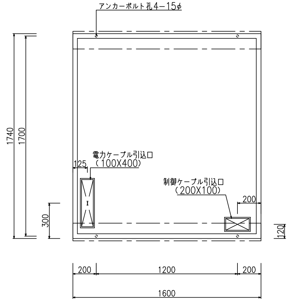
基礎図
