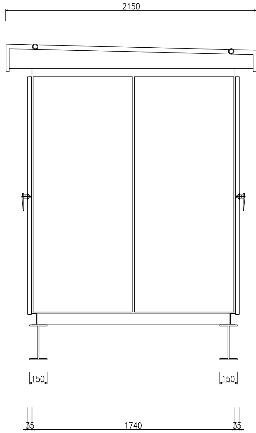
側面図
